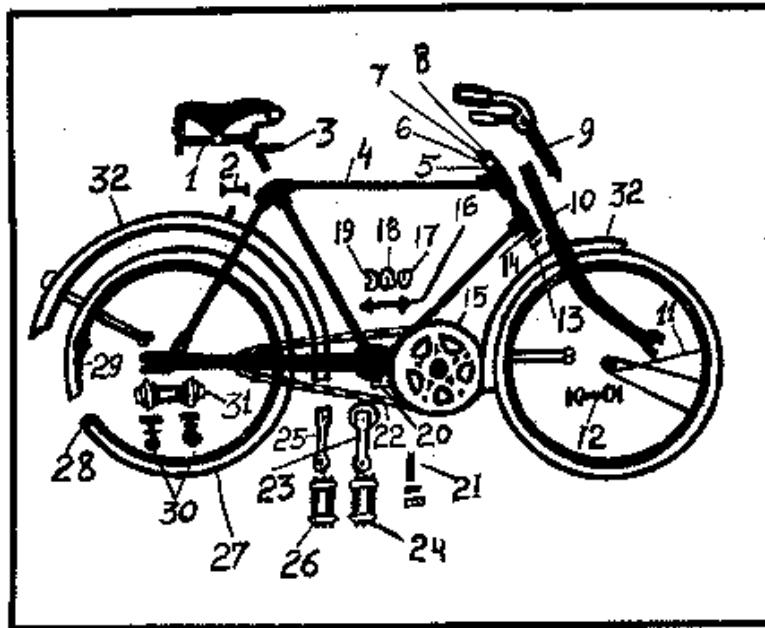
Рис. 50. Устройство велосипеда:
